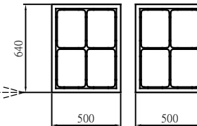
Standard (標準) Lower dust collector (下集塵器) Working area (工作範圍) : 500 x 640 mm
