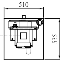
Dust collector EV-720 (集塵機 EV-720)
